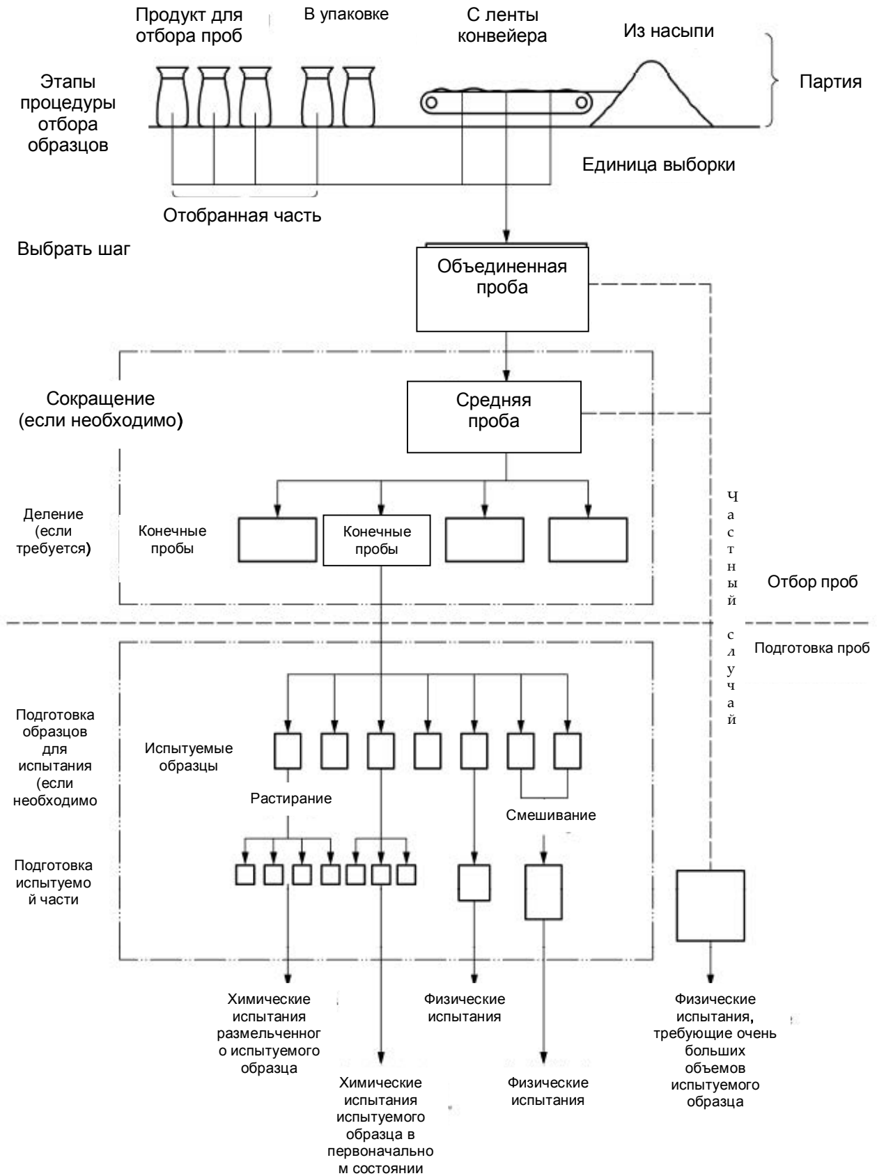
Рисунок 1 —Схема отбора проб твердых веществ
